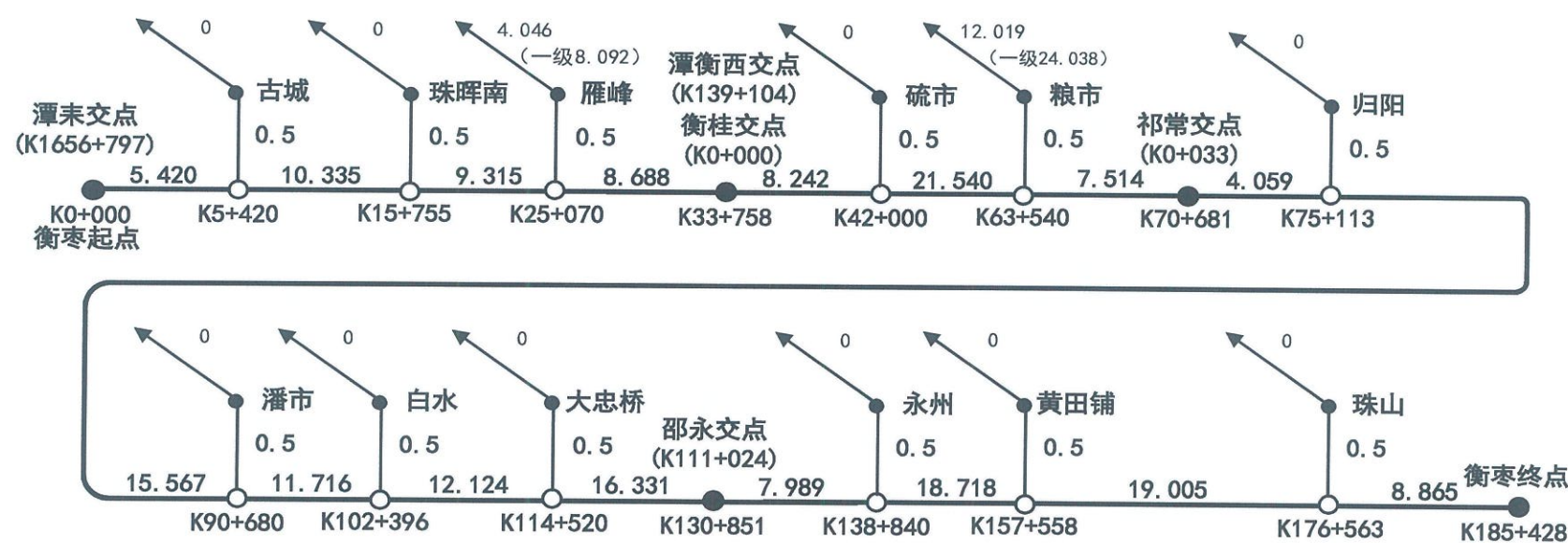
衡枣高速公路计费里程图式 (单位: Km)
